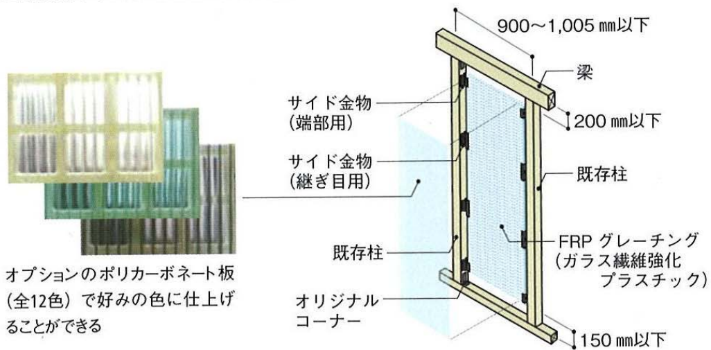
■構成図 (壁強さ倍率6.6kN/m)
